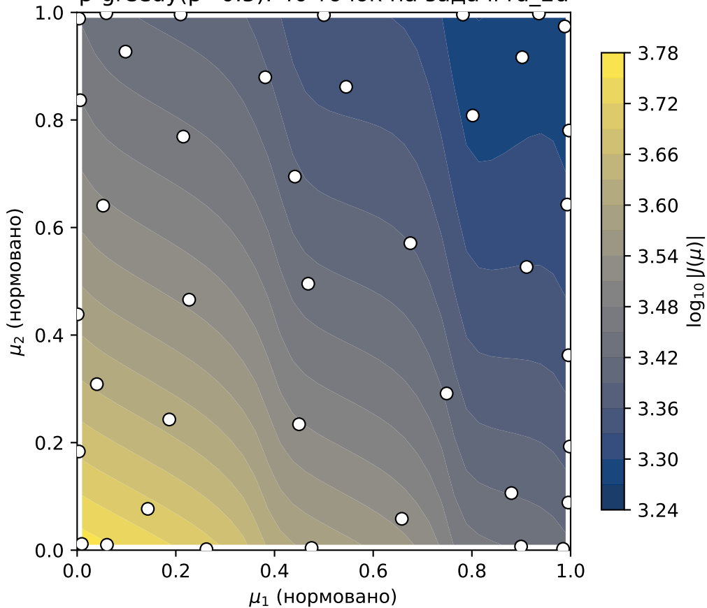
\beta -greedy( \beta=0.5 ): 40 точок на задачі rd_2d
